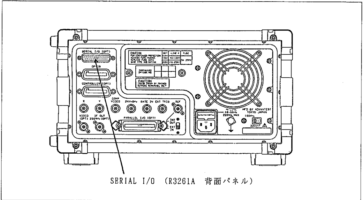
図 3 - 2 R3261/3361のRS-232C 通信ポート
