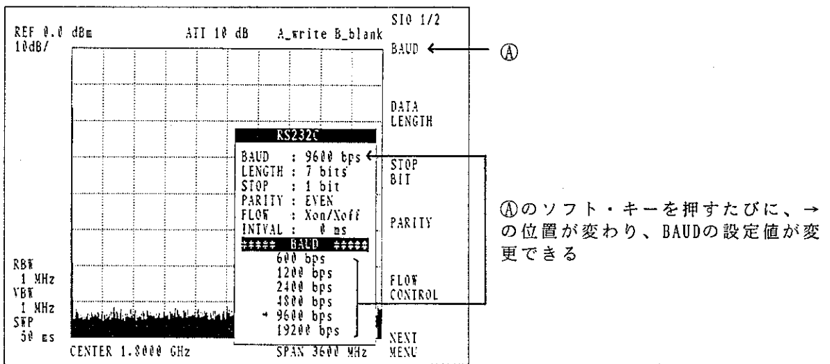
図 4 - 2 BAUDの設定画面
