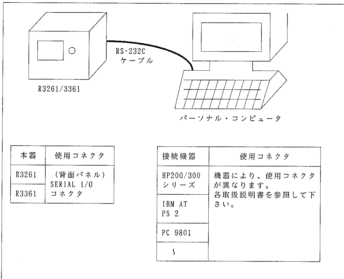
図 3 - 1 パーソナル・コンピュータの接続
