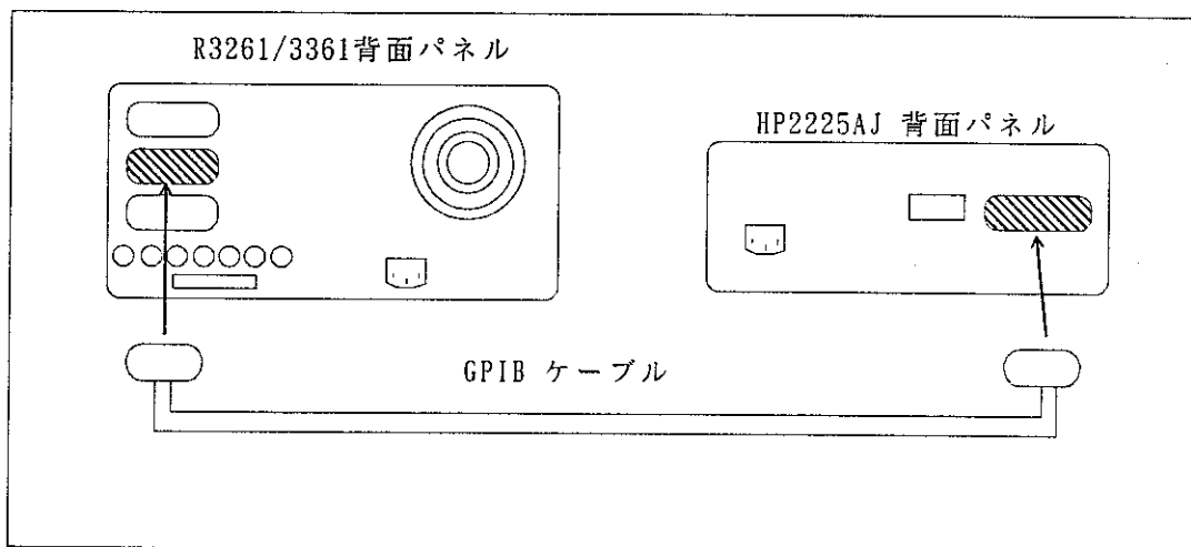
図 2 - 1 本器とプリンタの接続図
