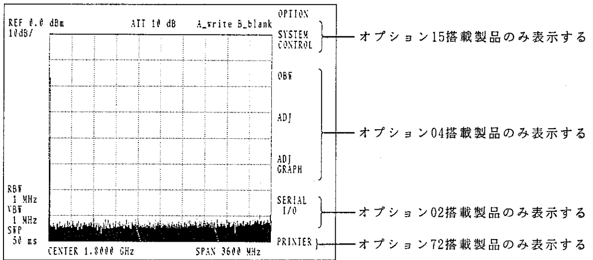
図 4 - 1 OPTION選択メニュー画面
