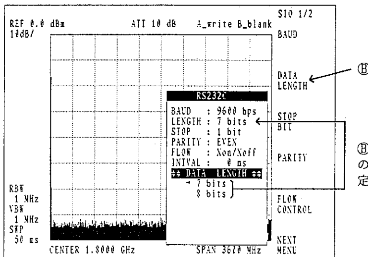
図 4 - 3 DATA LENGTH の設定画面
