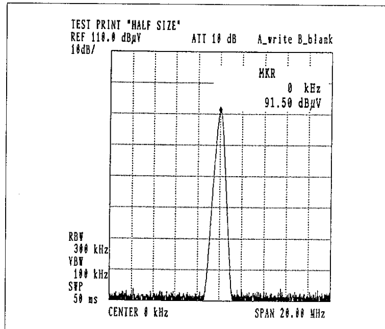
図 4 - 2 印刷サイズがHALFの場合
