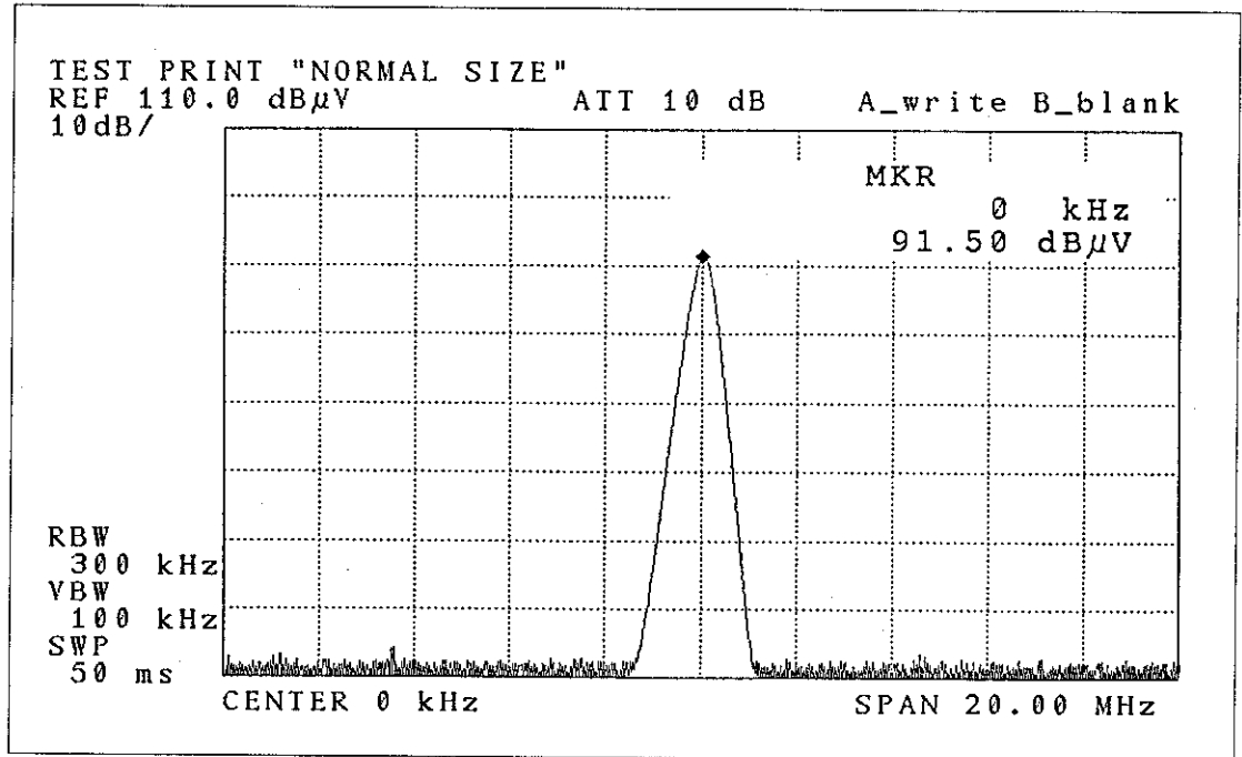
図 4 - 1 印刷サイズがNORMALの場合
