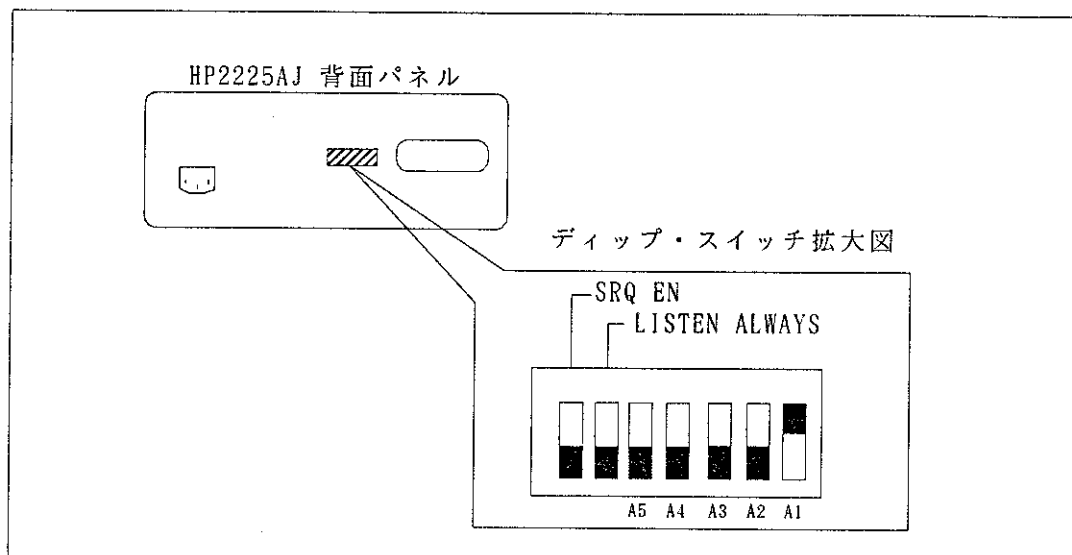
図 3 - 1 アドレス設定用ディップ・スイッチ
