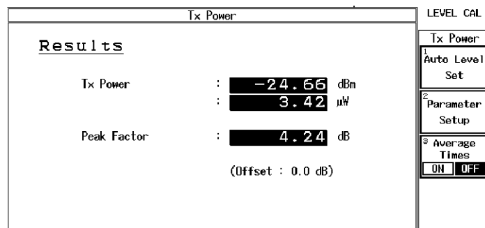
図 2-1 3GPP2 レベル・キャリブレーション機能を用いた 2 GHz の変調信号の設定例
