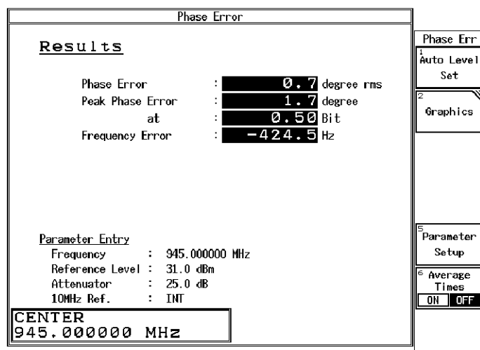
図 2-4 Phase Error 測定結果
