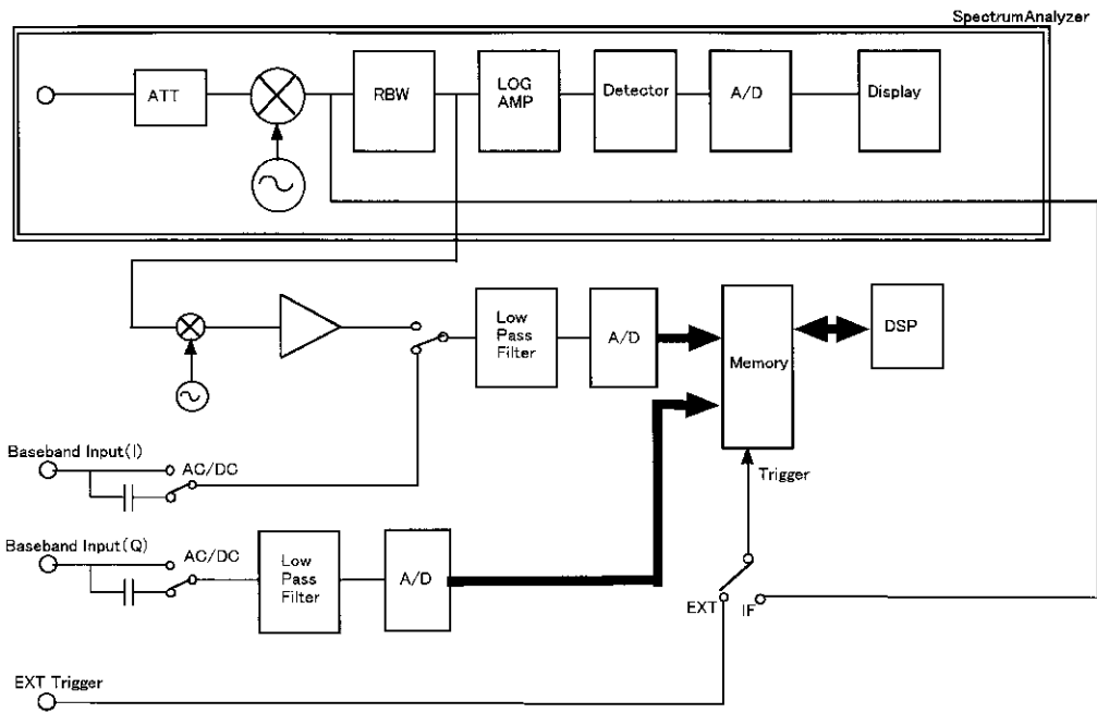
図 5-15 ブロック図
