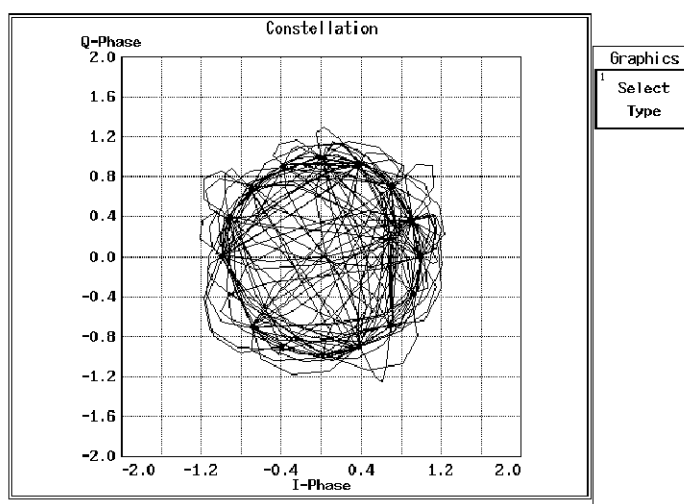
図 5-14 EDGE 信号 8PSK Constellation
