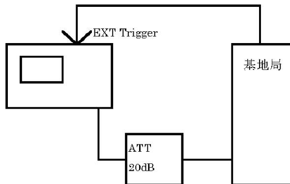
図 2-6 GSM 測定の接続
