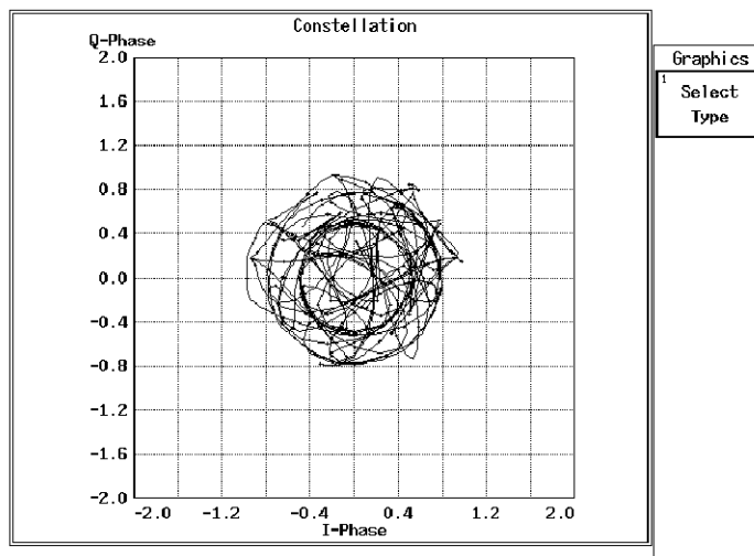
図 5-13 EDGE 信号の Constellation
