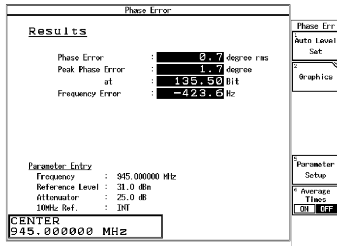
図 2-9 Phase Error 測定結果
