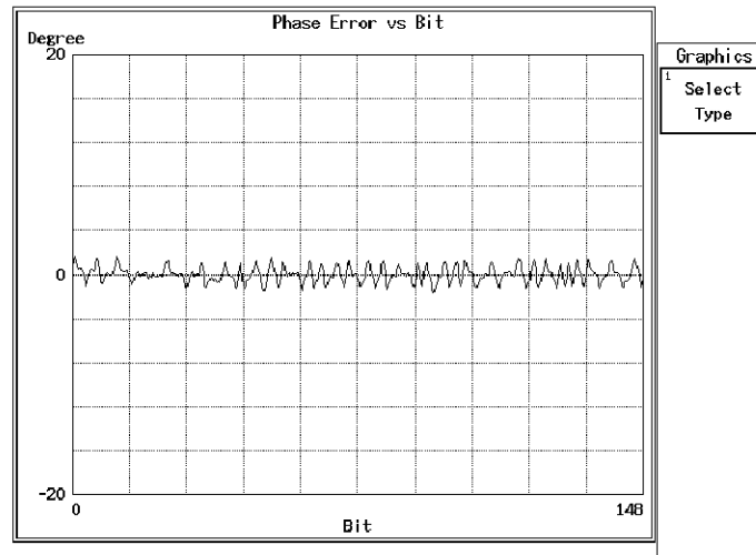
図 2-5 Phase Error vs Bit グラフ表示
