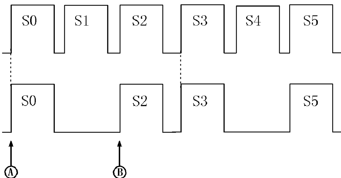
図 5-1 フレーム内に複数のバーストが存在する信号
