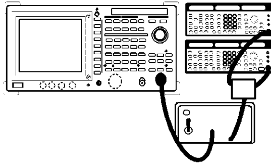
図 2-128 3次相互変調歪測定の接続
