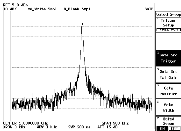
図 2-110 ゲーテッド・スイープによるバースト信号 (1 画面)
