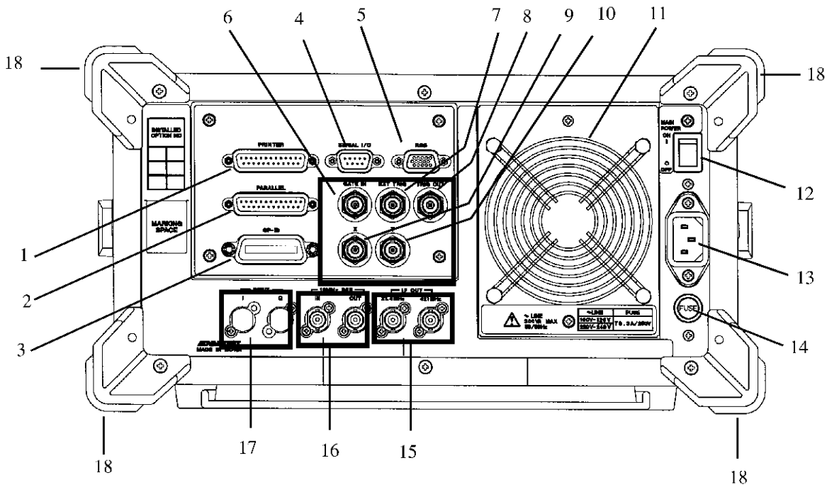
図 2-15 背面パネル
