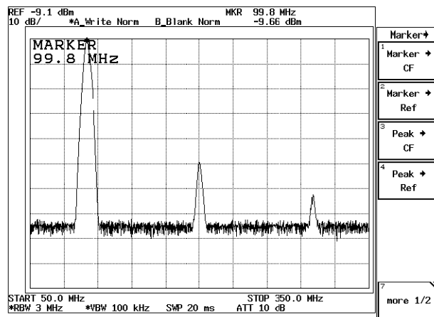
図 2-118 高調波のトレース
