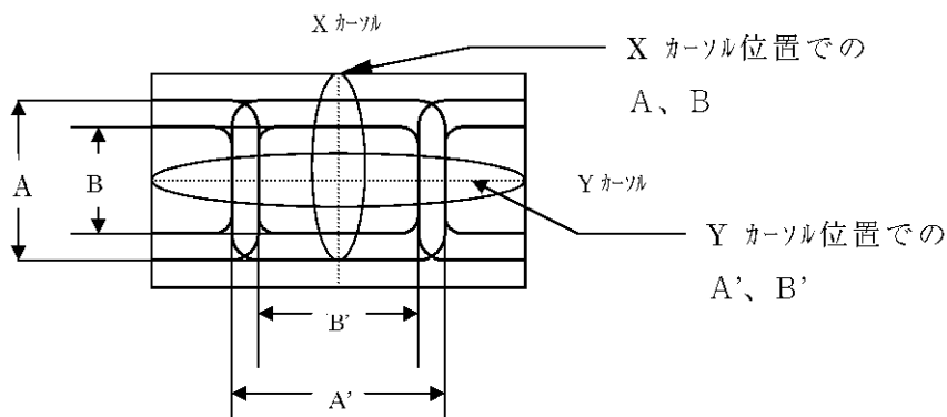
図 4-8 アイ開口率計算データ位置 (ウィンドウ表示 OFF 時)
