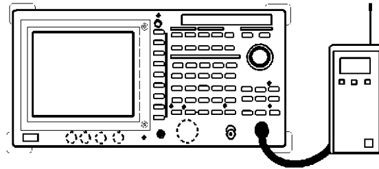
図 2-111 バースト信号測定接続
