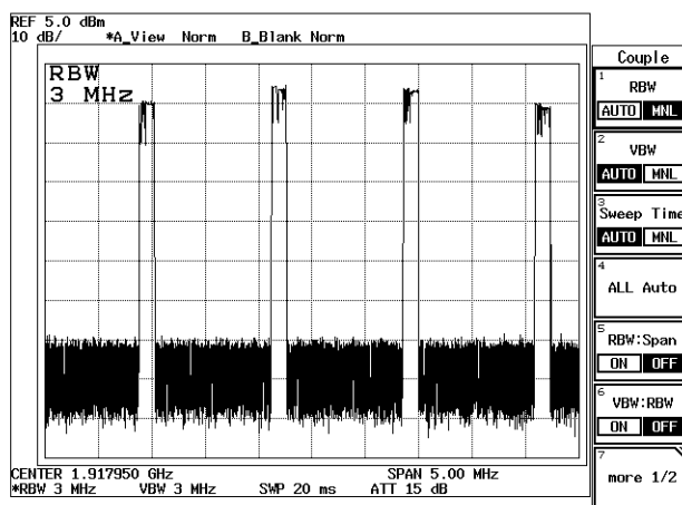
図 2-112 周波数ドメインにおけるバースト信号
