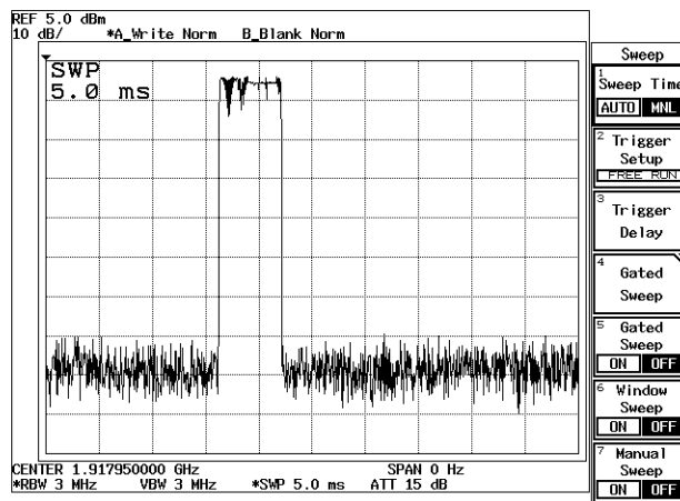
図 2-113 タイム・ドメインにおけるバースト信号
