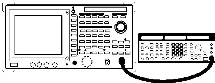
図 2-121 高調波測定の接続
