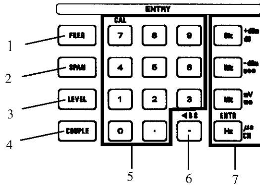
図 2-9 ENTRY セクションの説明
