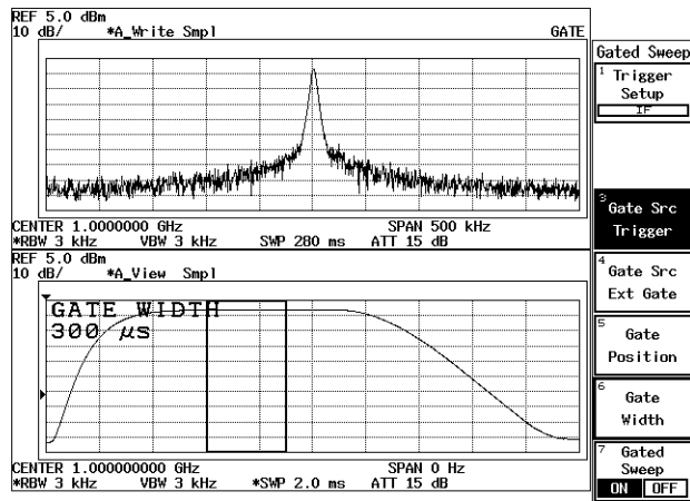
図 2-109 ゲーテッド・スイープによるバースト信号 (2 画面)
