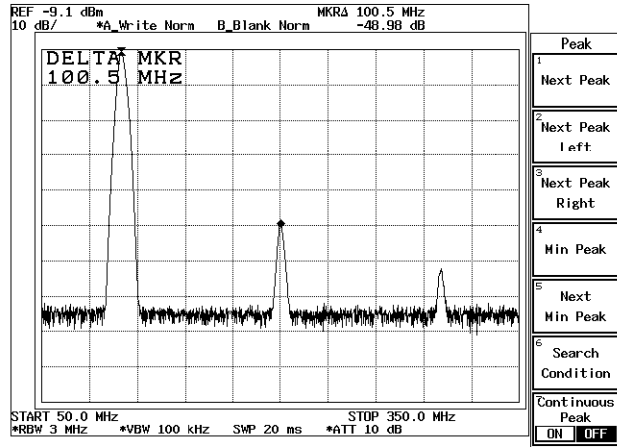
図 2-119 2次高調波
