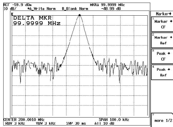
図 2-126 2 次高調波
