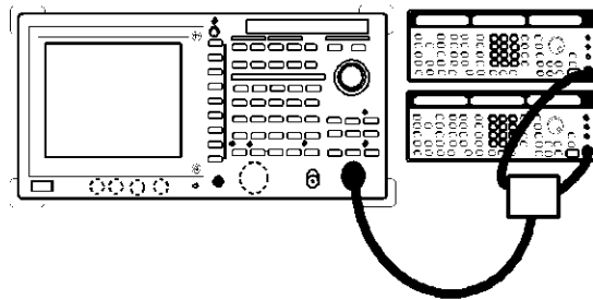
図 2-37 2 信号の分離測定への接続
