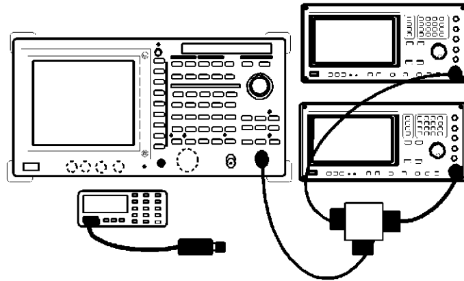
図 1-13 2 信号 3 次歪の測定の接続
