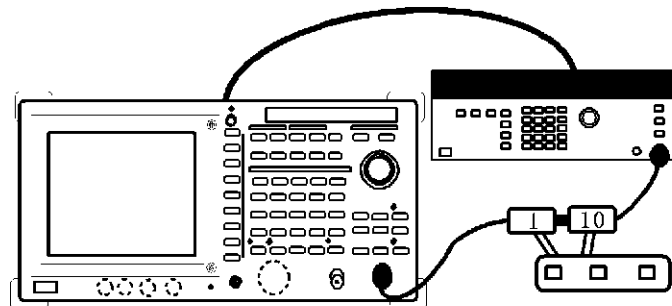
図 1-8 スケール表示確度の測定の接続
