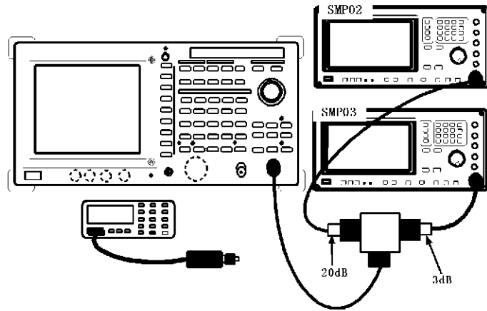
図 1-11 利得圧縮の測定の接続
