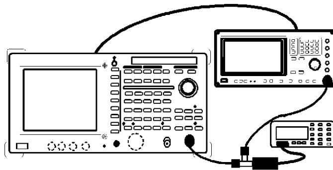
図 1-14 イメージ／マルチプル／バンド外応答測定接続
