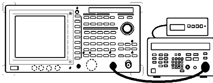
図 1-1 基準周波数確度の測定の接続
