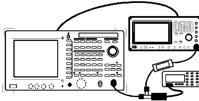
図 1-12 2次高調波歪の測定接続
