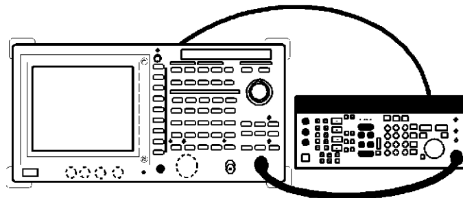
図 1-9 信号純度の測定接続
