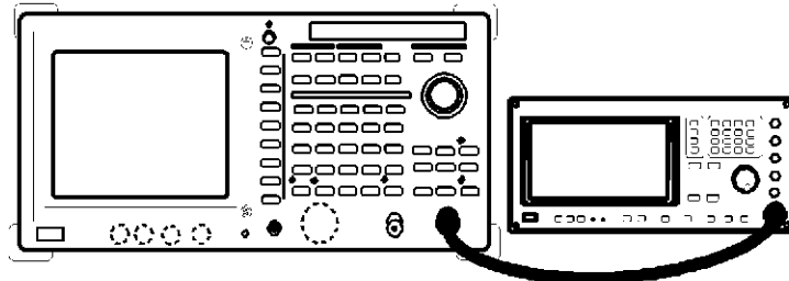
図 1-6 アッテネータ切り換え確度の測定の接続
