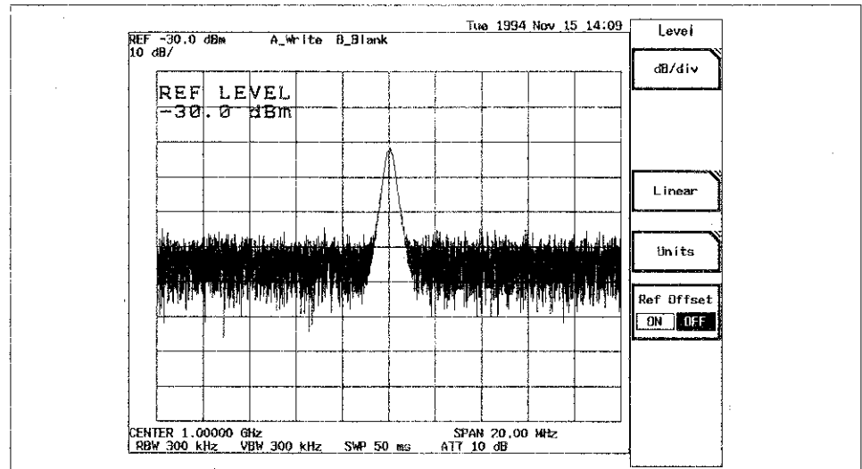
図 7 - 7 VBW=300kHz
