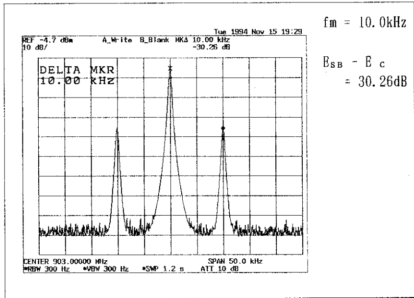
図 5 - 9 変調周波数が高く、変調指数が小さいAM波
