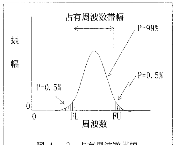
図 A - 3 占有周波数帯幅
