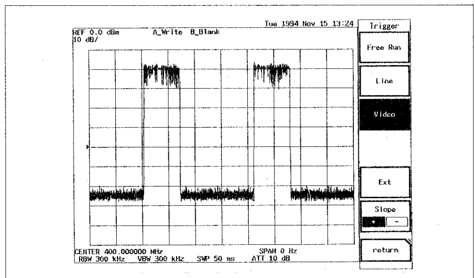
図 7 - 20 画面上に表示された波形でトリガをかける
