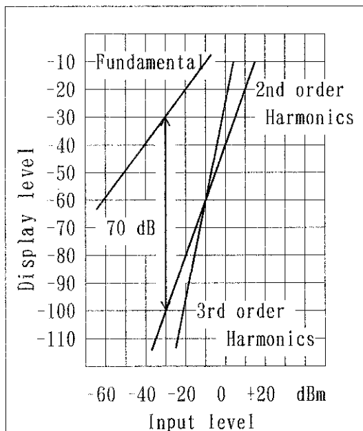
図 A - 4 スプリアス・レスポンス
