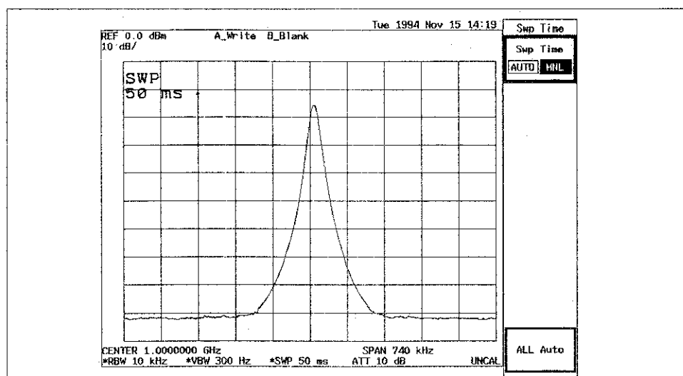
図 7 - 22 SWP=50ms
