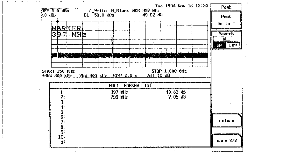
図 7 - 17 Up設定時
