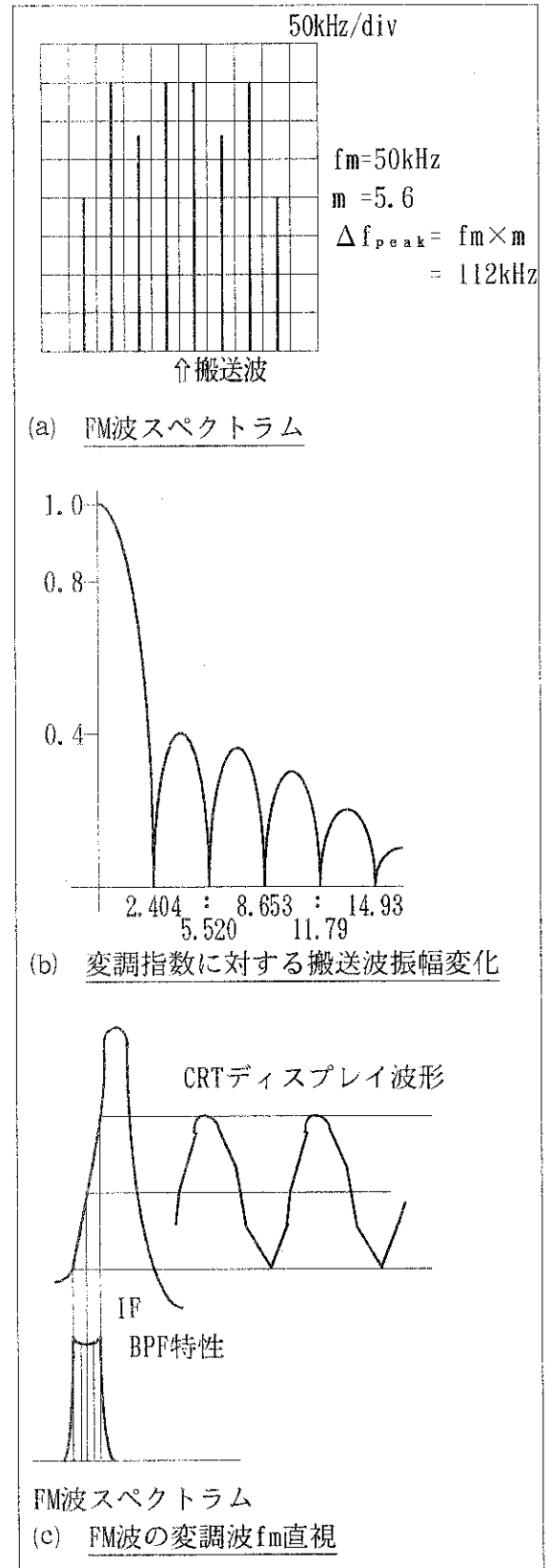
図 5 - 11 FM 信号の測定
