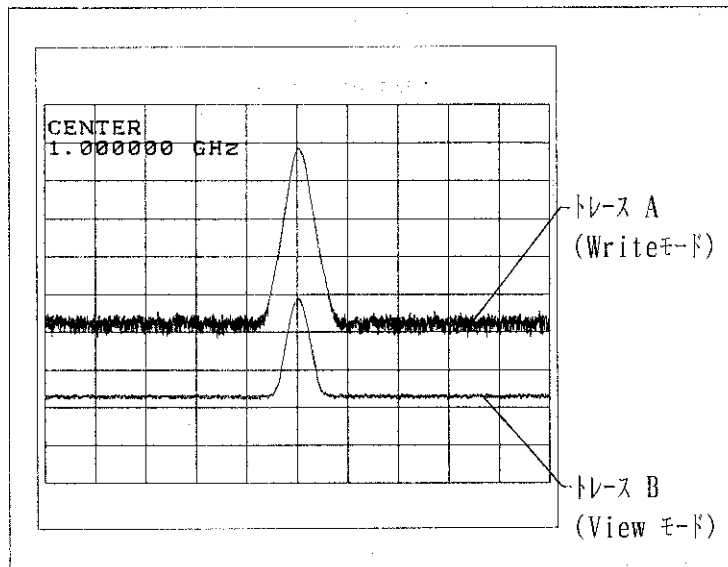
図 7 - 10 Write モードとViewモード
