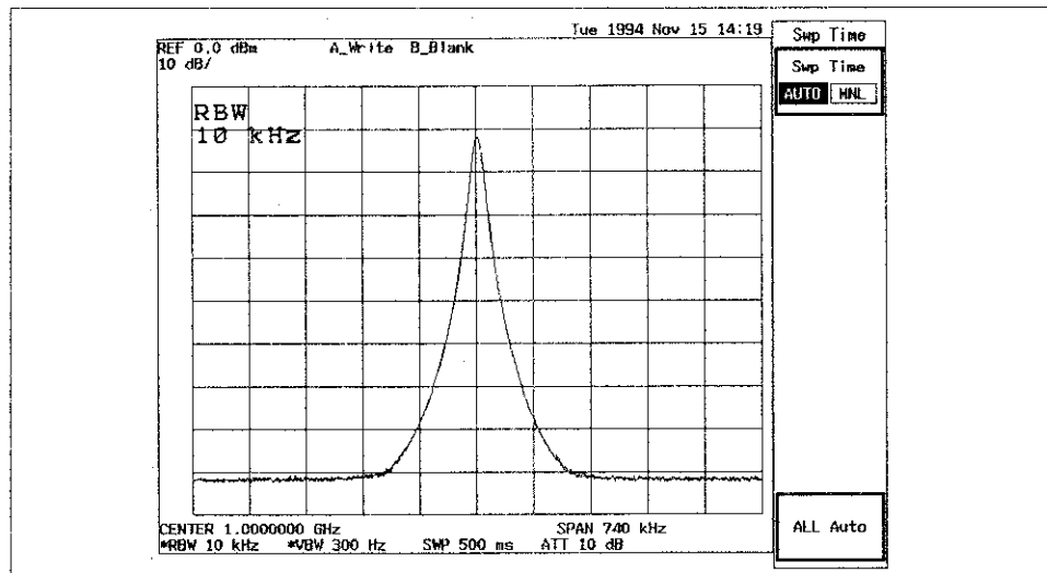
図 7 - 21 SWP=AUTO(500ms)
