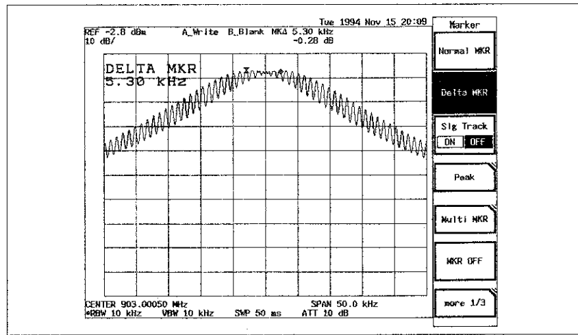
図 5 - 19 \Delta f_{\text{peak}} が小さいFM波
