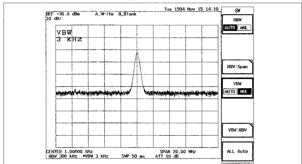
図 7 - 8 VBW=3kHz
