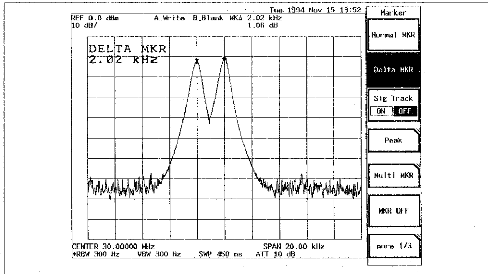
図 7 - 6 RBW : 2 信号として分離できる最大のIFバンド幅
