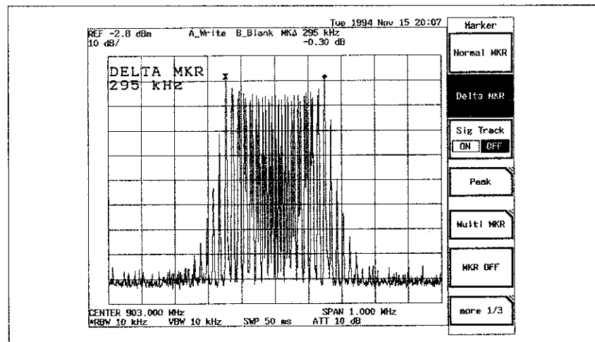
図 5 - 20 \Delta f_{\text{peak}} が大きいFM波
