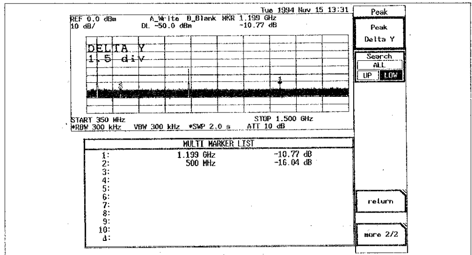
図 7 - 18 Low 設定時
