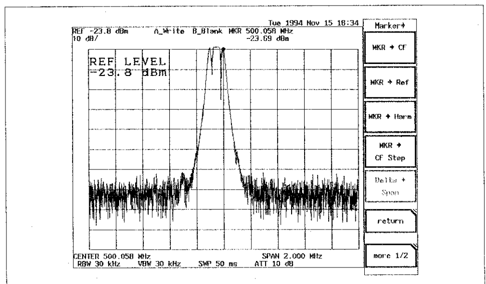
図 3 - 18 MKR⇒REF機能
