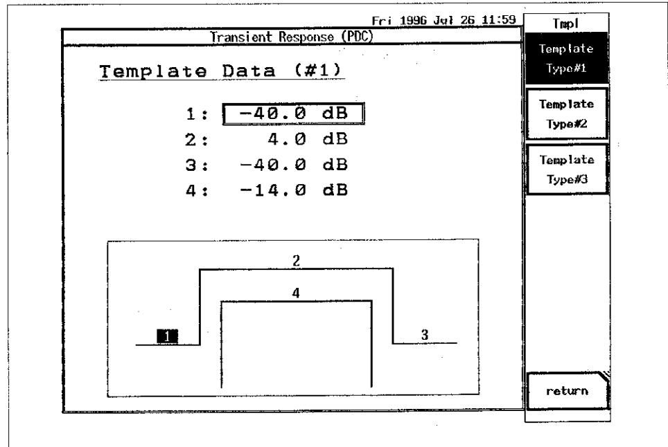
図1-9 Userテンプレート登録画面
