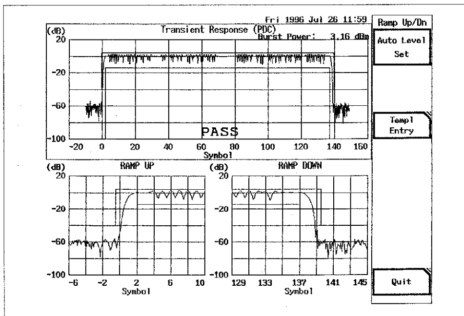
図1-8 Ramp UP/DOWN測定例
