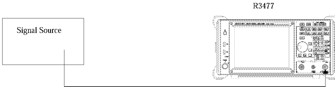
図 4-14 Ramp 測定の接続図
