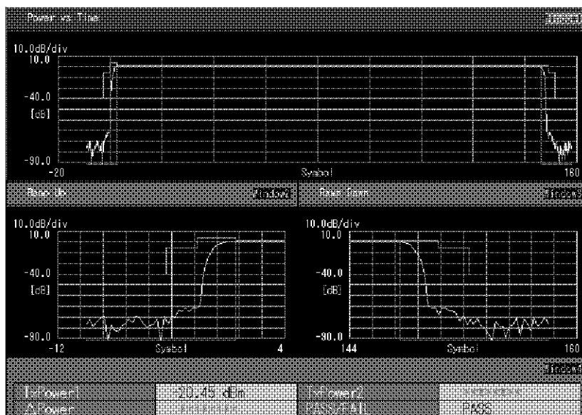
図 4-10 Power vs Time 測定結果
