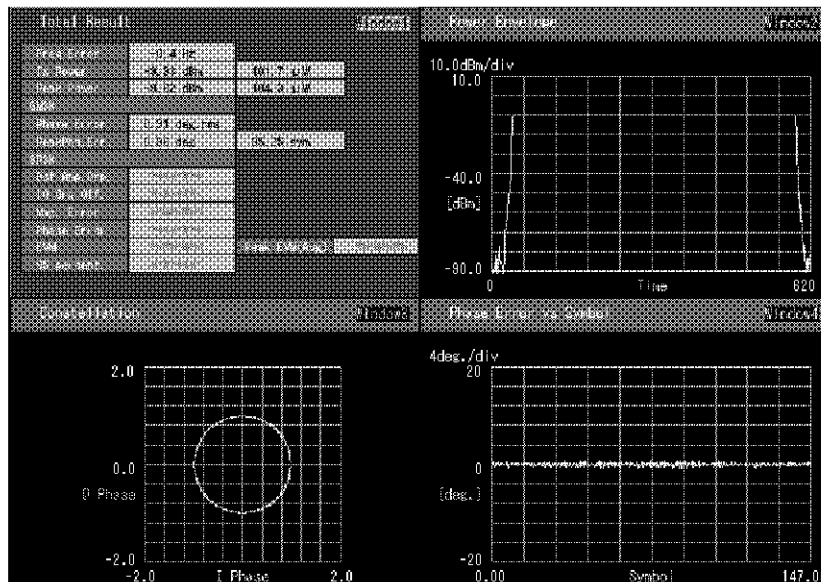
図 4-4 変調精度測定結果
