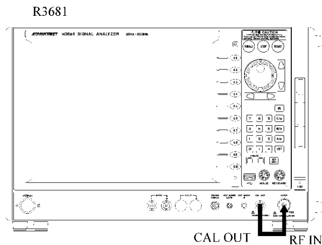
図 7-1 信号源の接続図
