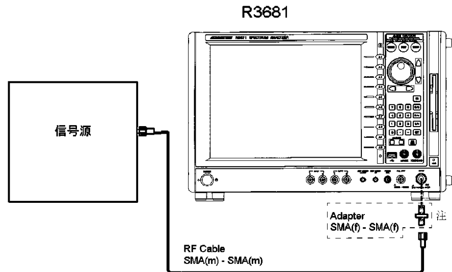
図 4-5 Power vs Time 接続図
