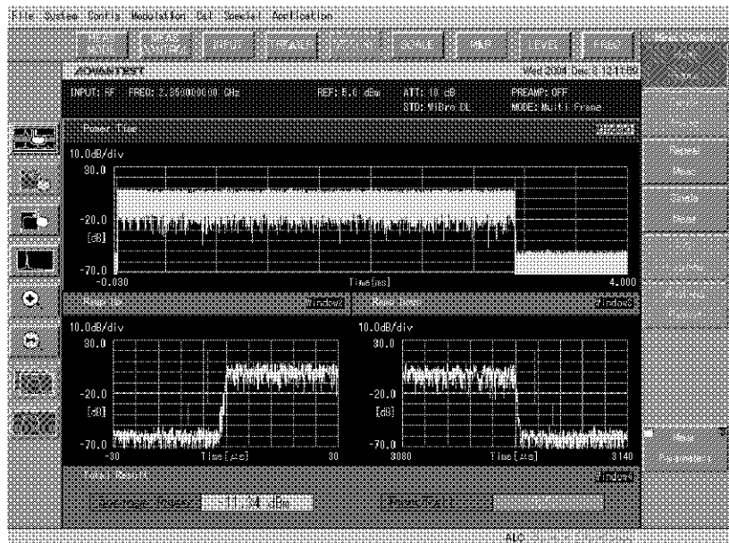
図 4-28 Ramp 測定例
