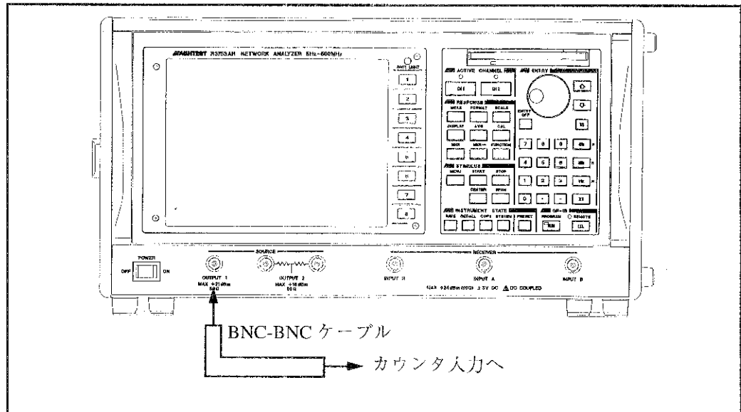
図 5-1 周波数精度と範囲
