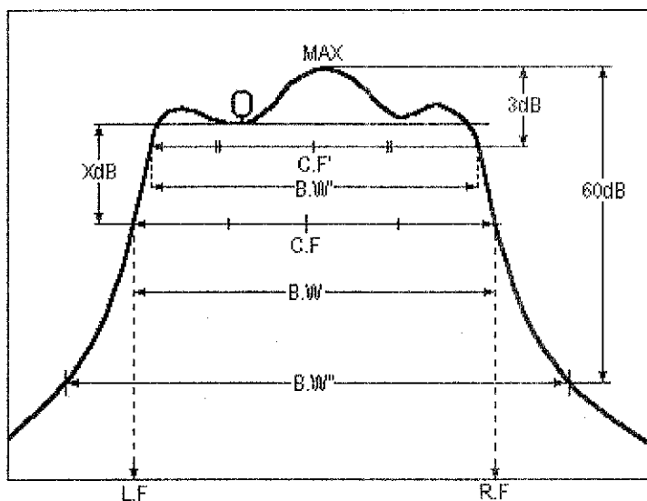
図 4-3 バンドパス・フィルタ解析 / アクティブ・マーカ基準
