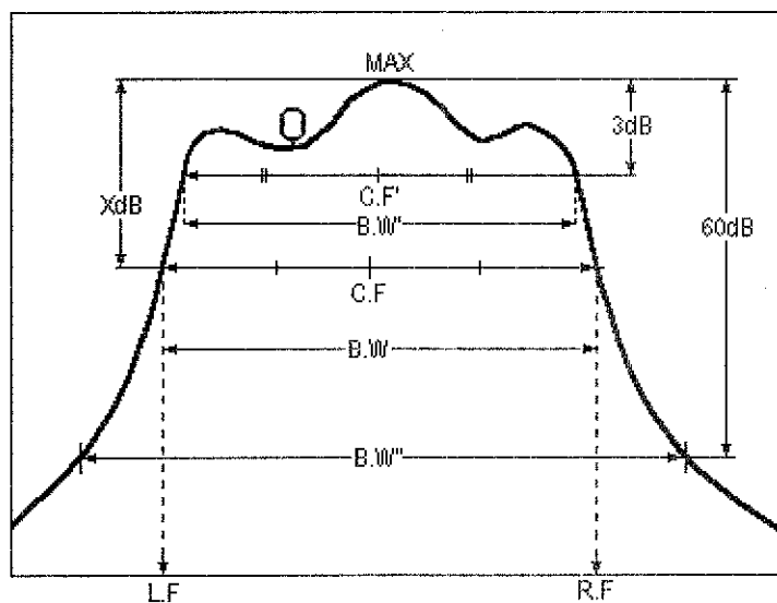
図 4-2 バンドパス・フィルタ解析 / MAX 基準
