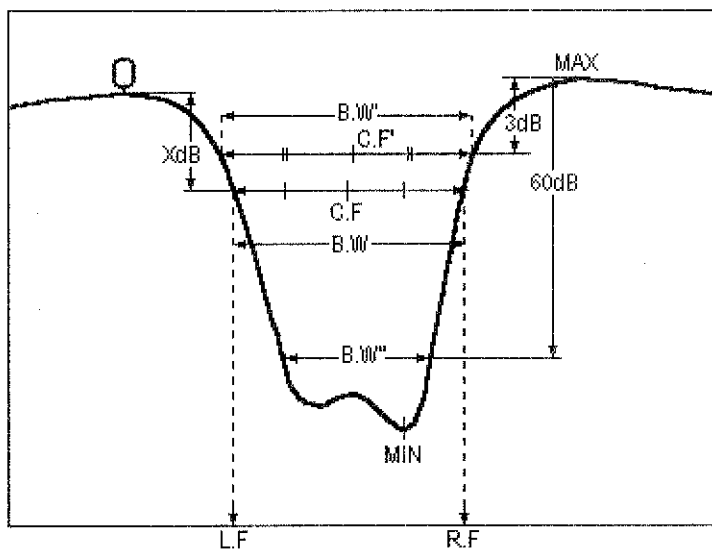
図 4-6 ノッチ・フィルタ解析 / アクティブ・マーカ基準
