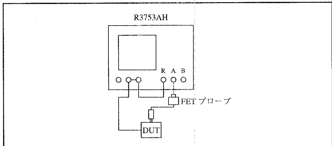
図 1-6 FET プロープの接続 (比測定の場合)
