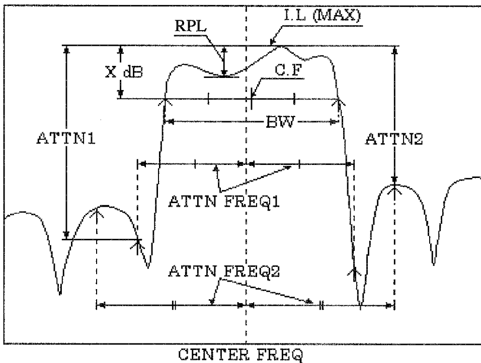
<CDMA IF フィルタ振幅解析例>
