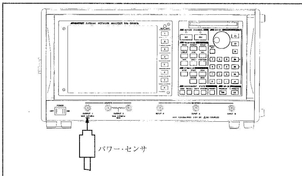
図 5-2 出力レベル精度とフラットネス
