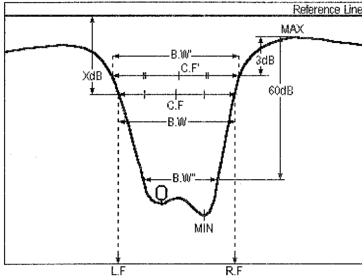
図 4-7 ノッチ・フィルタ解析 / リファレンス・ライン基準
