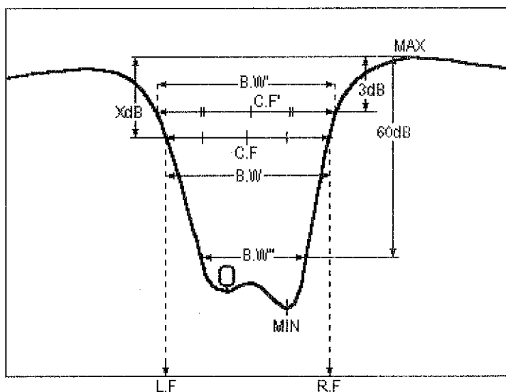
図 4-5 ノッチ・フィルタ解析 / MAX 基準
