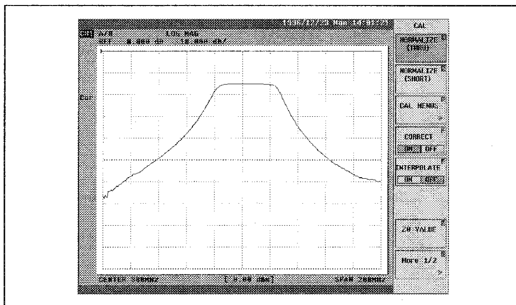
図 3-84 リミット・ライン測定の実行前画面
