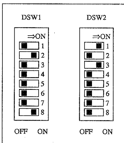
図 4-11 デイック・スイッチの設定
