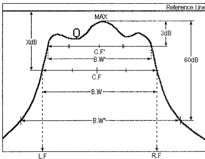
図 4-4 バンドパス・フィルタ解析 / リファレンス・ライン基準
