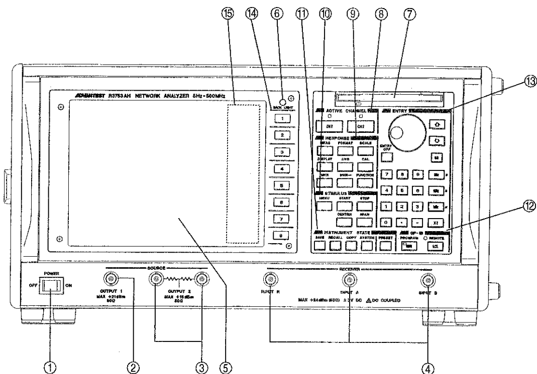
図 2-1 正面パネルの説明 (R3753AH)
