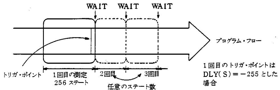
図-6 TRACE THEN WAIT によるステート解析
