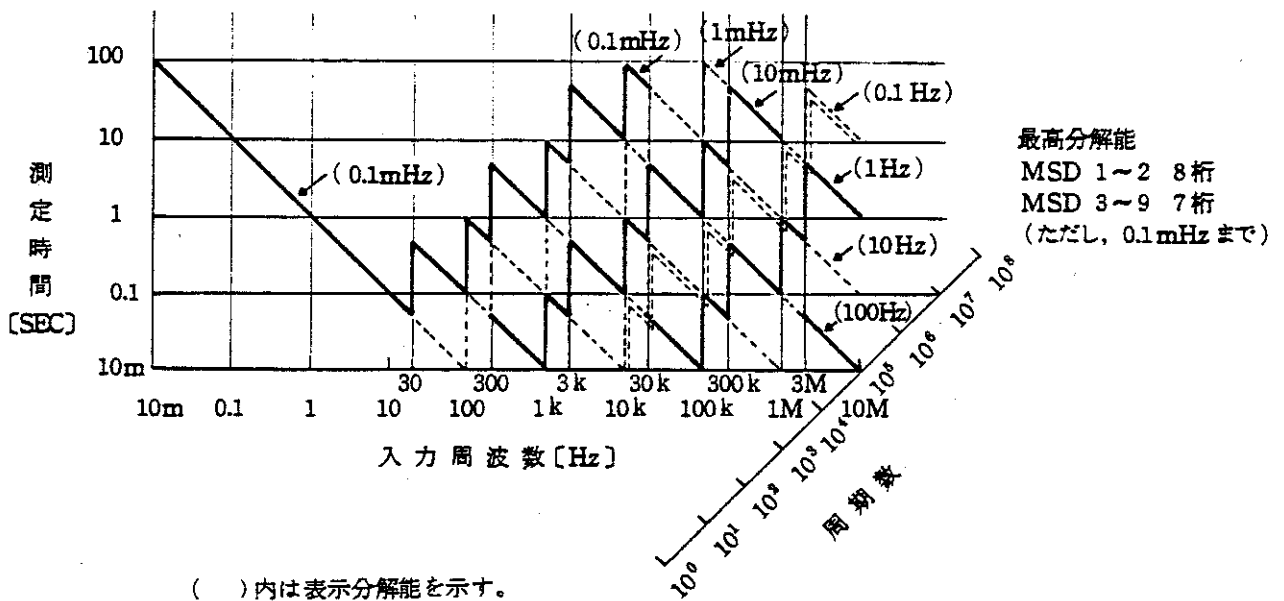
図 2-1 A入力 (Low) レシプロカル方式の入力周波数に対する測定時間, 分解能, 周期数
