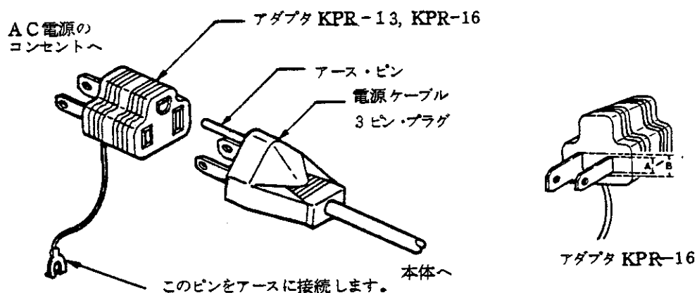
図3-1 電源ケーブルのプラグとアダプタ
