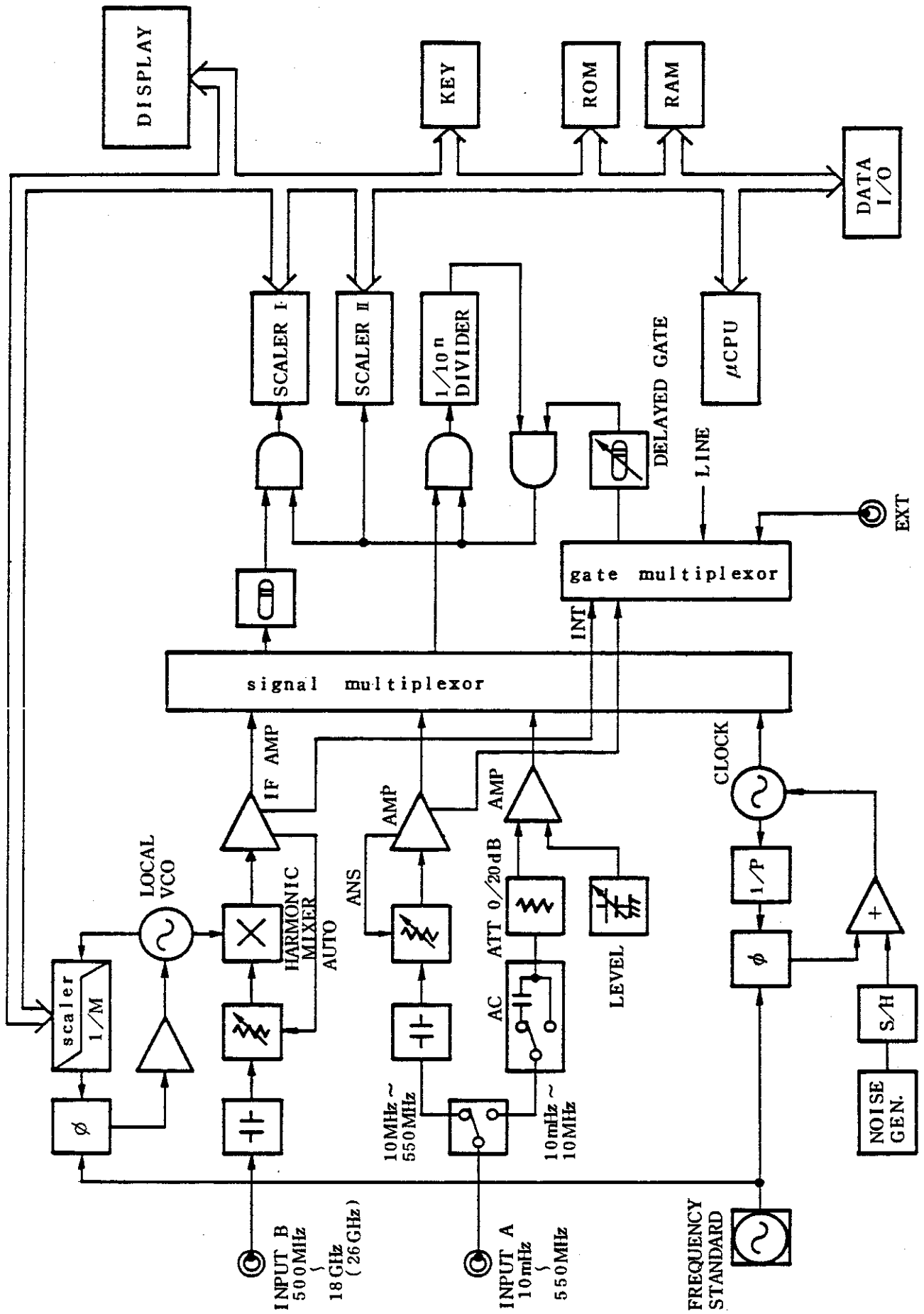
図 6-1 TR5212P/13P ブロック・ダイアグラム
