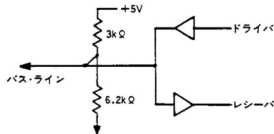
図 7-2 信号線の終端
