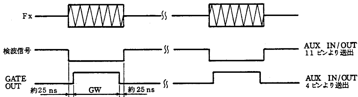
図 3-6 バースト波測定
