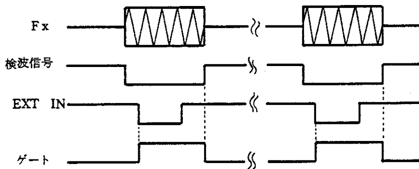
図 3-9 EXT STARTモード
